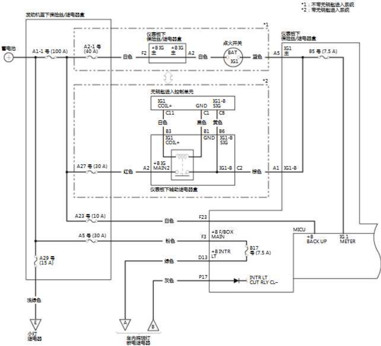
车内照明灯电路图
